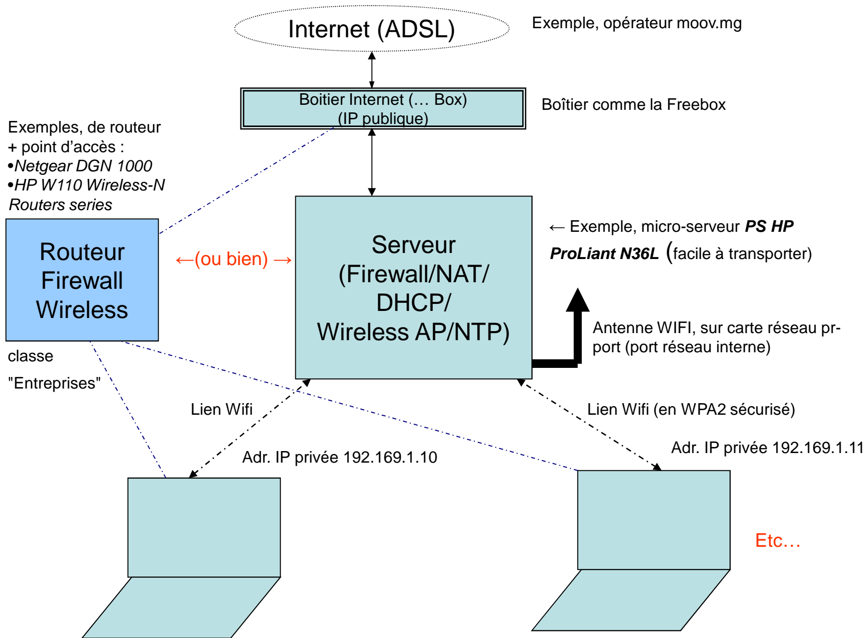
Architecture informatique WIFI pour salle informatique du lycée A...
